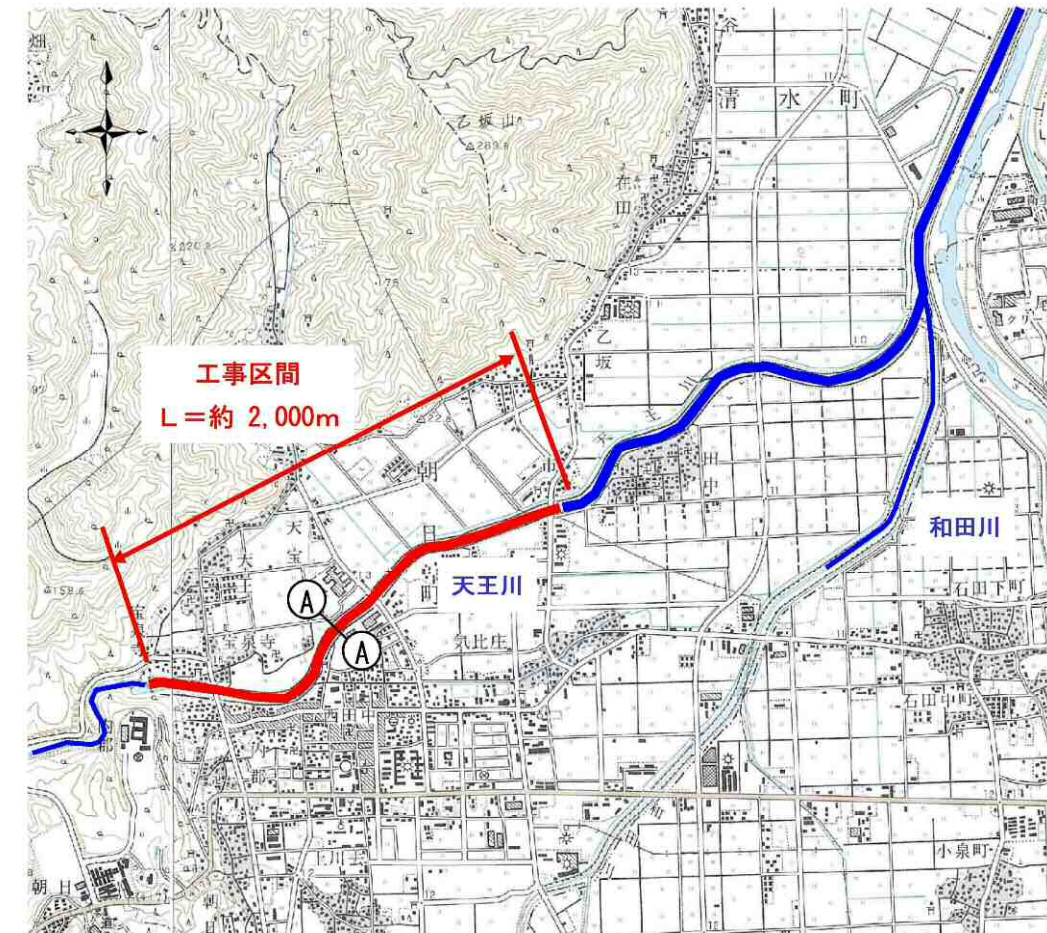
図 5.16 平面図
