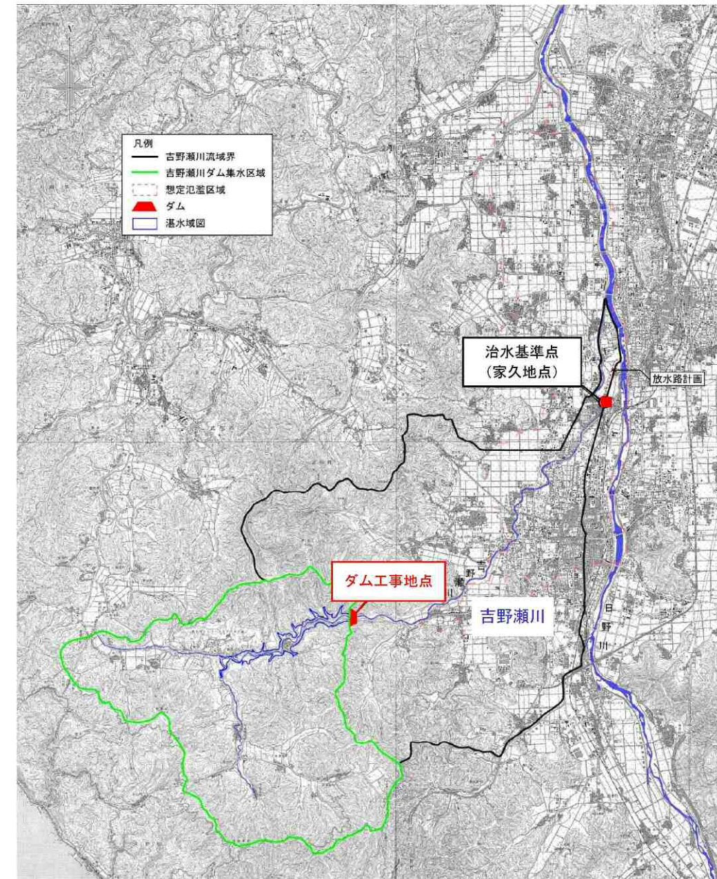
図 5.20 ダム位置図
