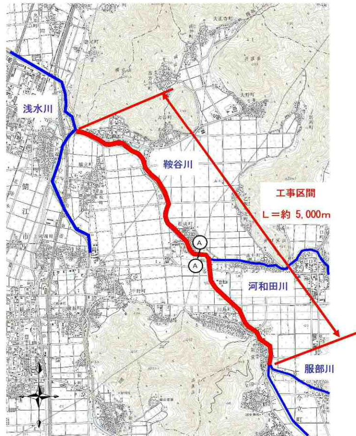
図 5.13 平面図
