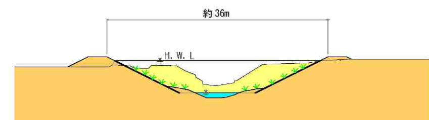
図 5.11 横断面図 (イメージ)
