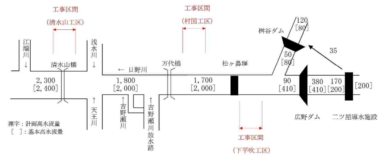
図 5.2 計画流量配分図
