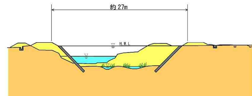
図 5.14 横断面図 (イメージ)
