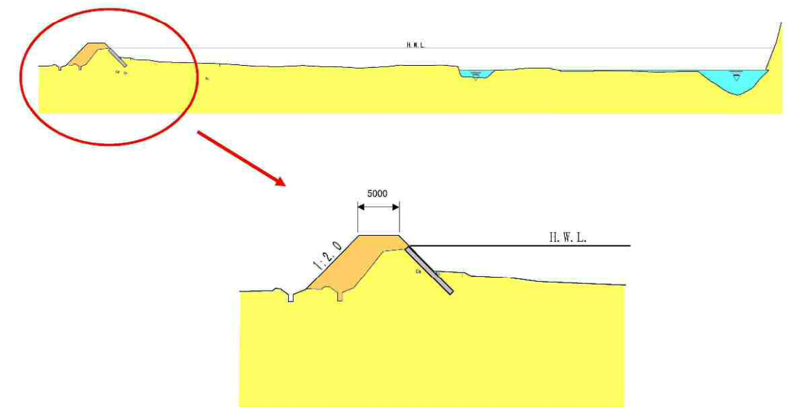
図 5.8 横断面 (イメージ)
