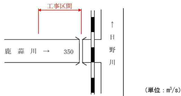
図 5.31 計画流量配分図
