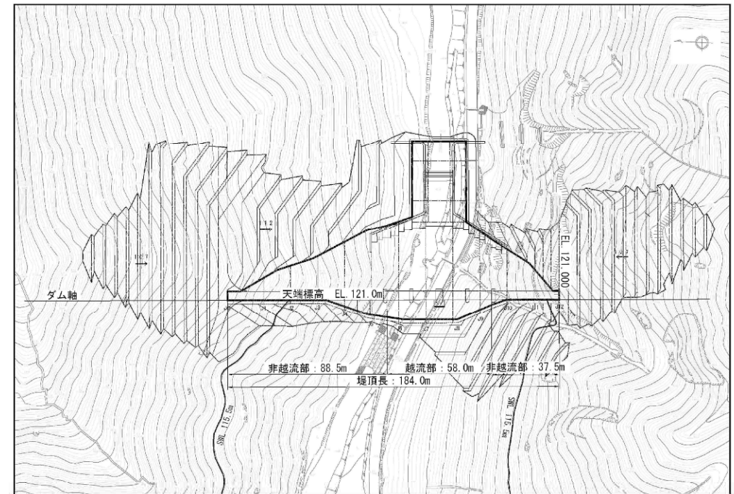
図 5.21 平面図
