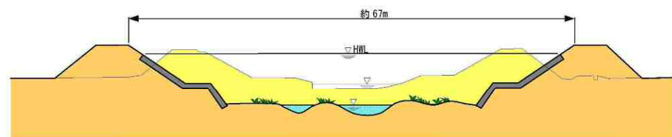
図 5.14 横断面図 (イメージ)
