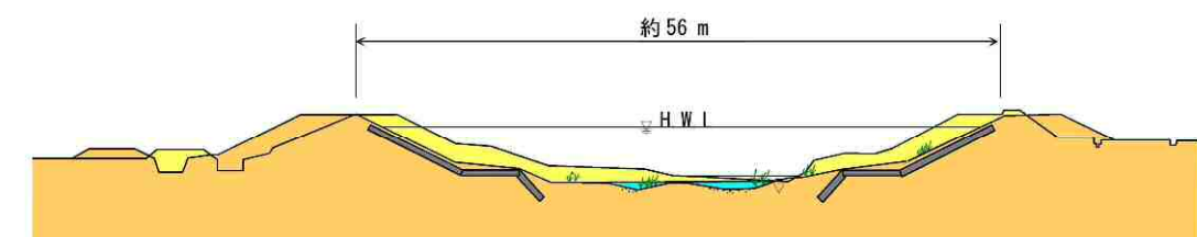
図 5.17 横断面 (イメージ)
