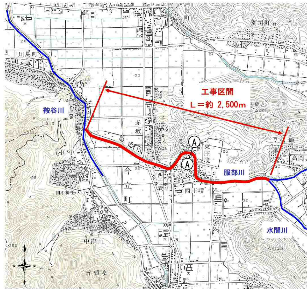
図 5.19 平面図
