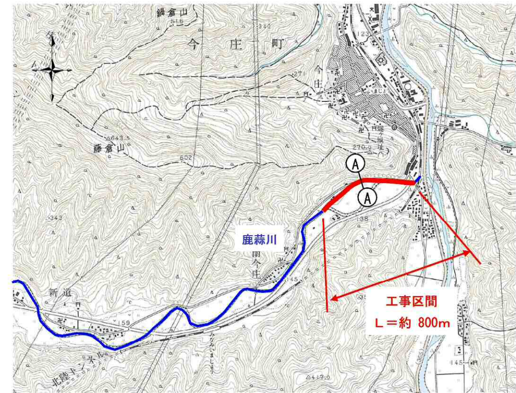
図 5.26 平面図
