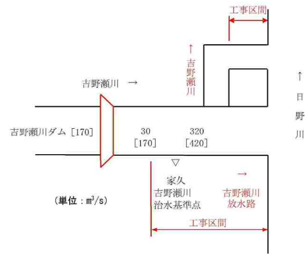
図 5.24 計画流量配分図
