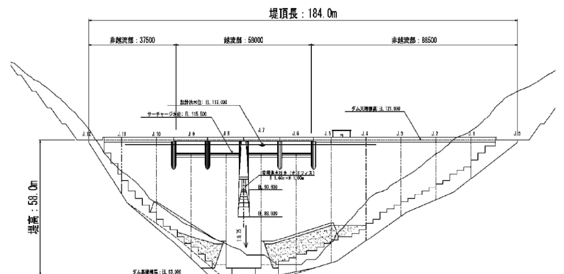
図 5.22 下流面図
