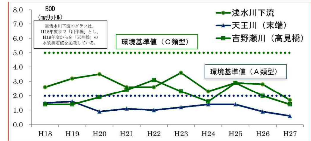
図 3.2 支川の水質 (BOD 75%値) の推移
