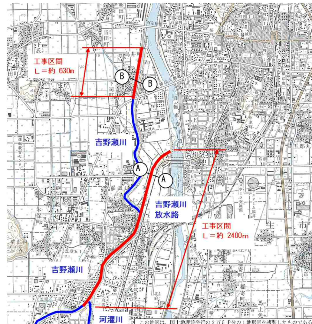
この地図は、国土地理院発行の2万5千分の1地形図を複製したものである。 図 5.23 平面図
