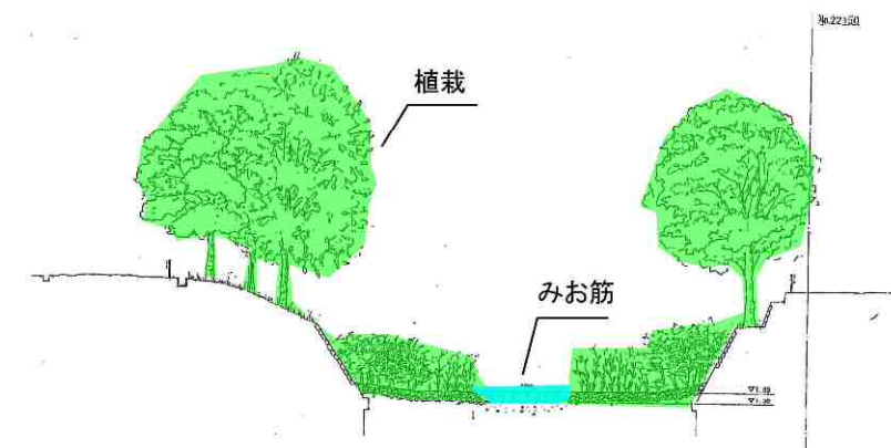
図 5.29 横断面図 (イメージ)
