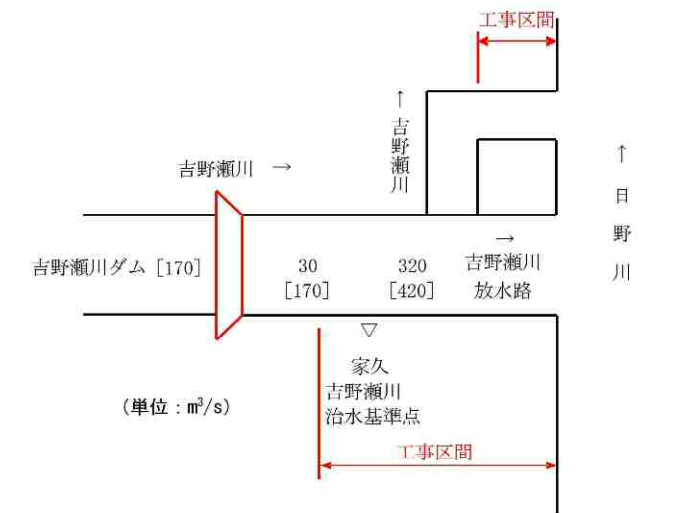
図 5.18 計画流量配分図
