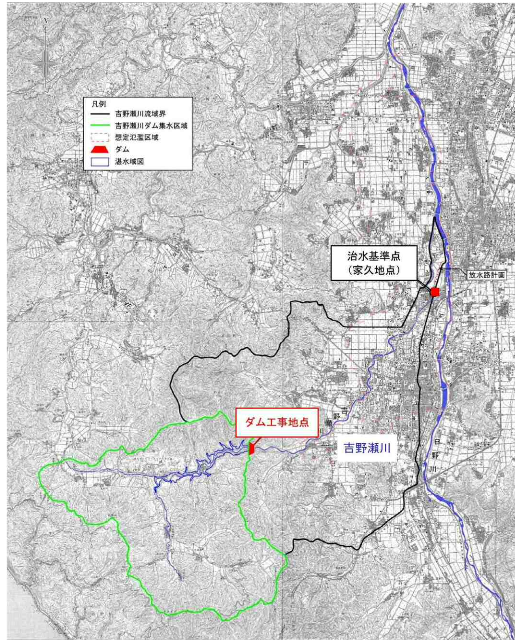
図 5.26 ダム位置図
