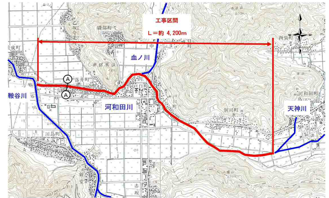
図 5.13 平面図
