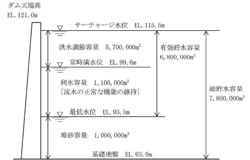
図 5.19 ダム容量配分図
