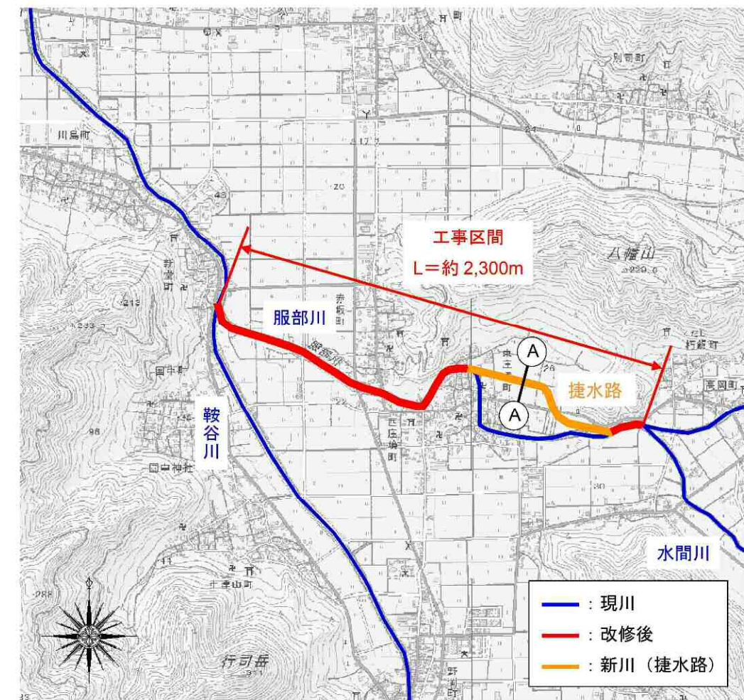
図 5.19 平面図
