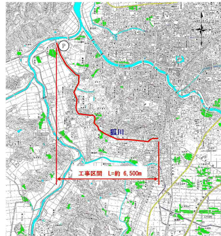
図 5.28 平面図
