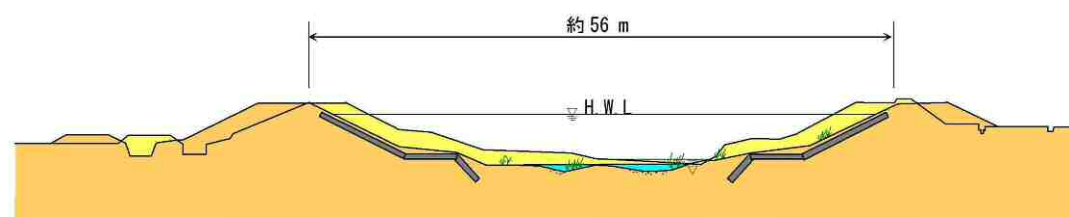
図 5.23 横断面 (イメージ)
