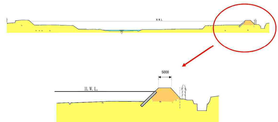
図 5.6 横断面図 (イメージ)
