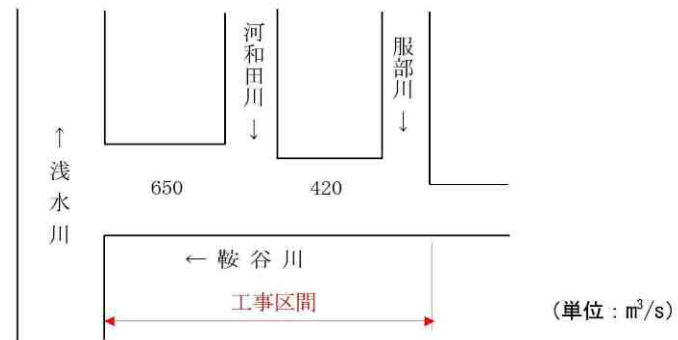
図 5.12 計画流量配分図
