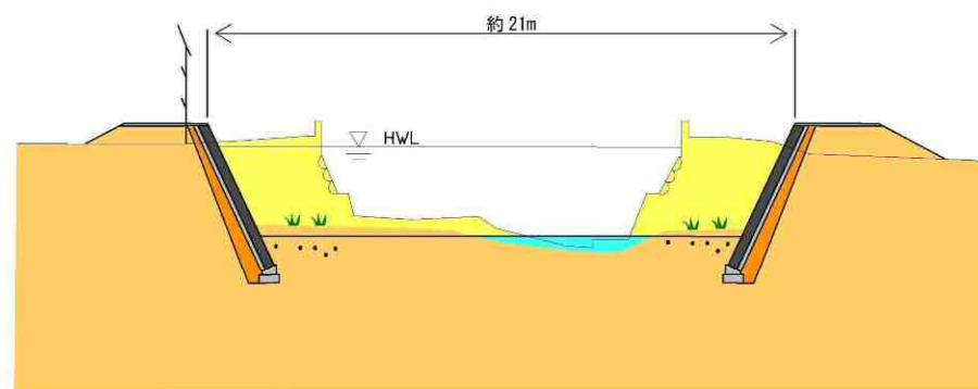
図 5.20 横断面 (イメージ)
