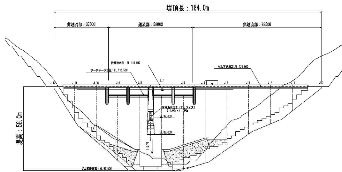
図 5.28 下流面図
