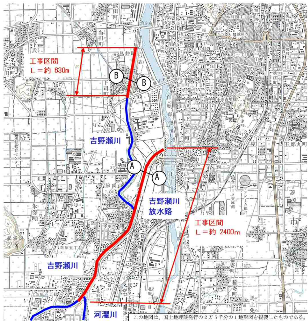
この地図は、国土地理院発行の2万5千分の1地形図を複製したものである。 図 5.29 平面図
