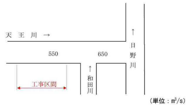
図 5.21 計画流量配分図
