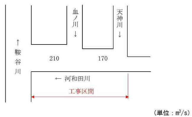
図 5.12 計画流量配分図
