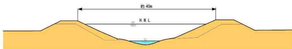
図 5.30 横断面図 (イメージ)
