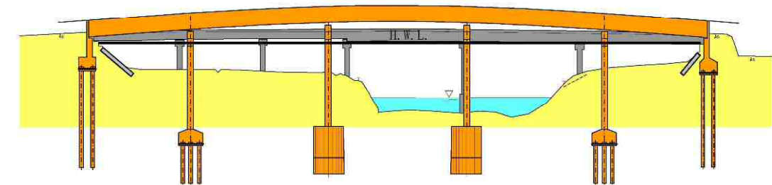
図 5.4 横断面 (イメージ)
