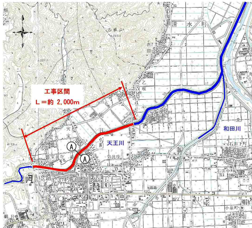
図 5.22 平面図
