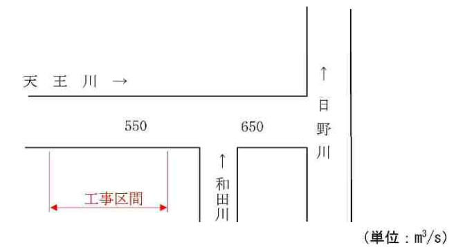
図 5.15 計画流量配分図
