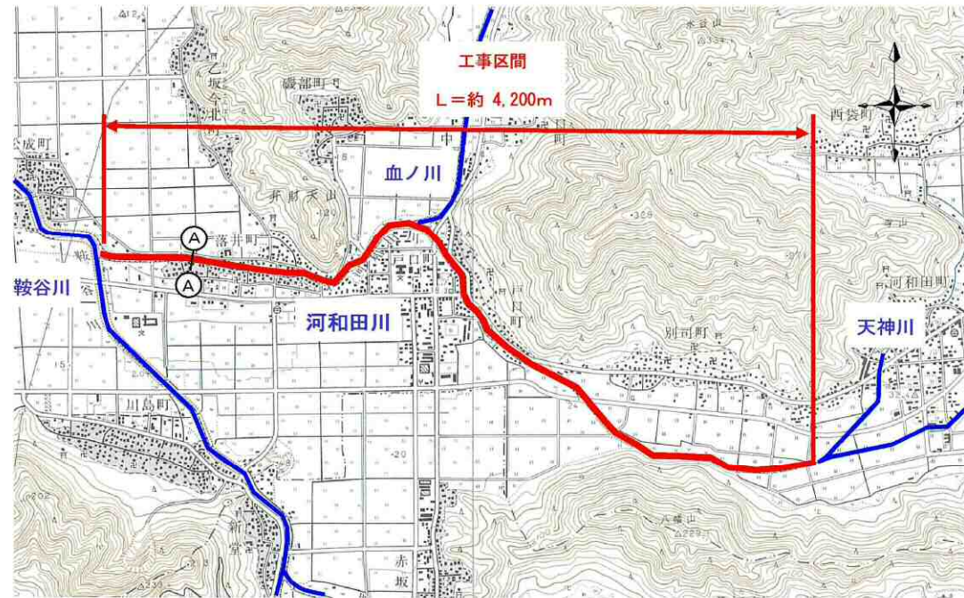
図 5.16 平面図
