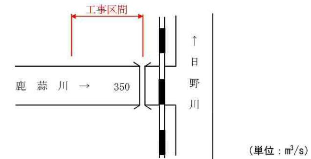
図 5.25 計画流量配分図
