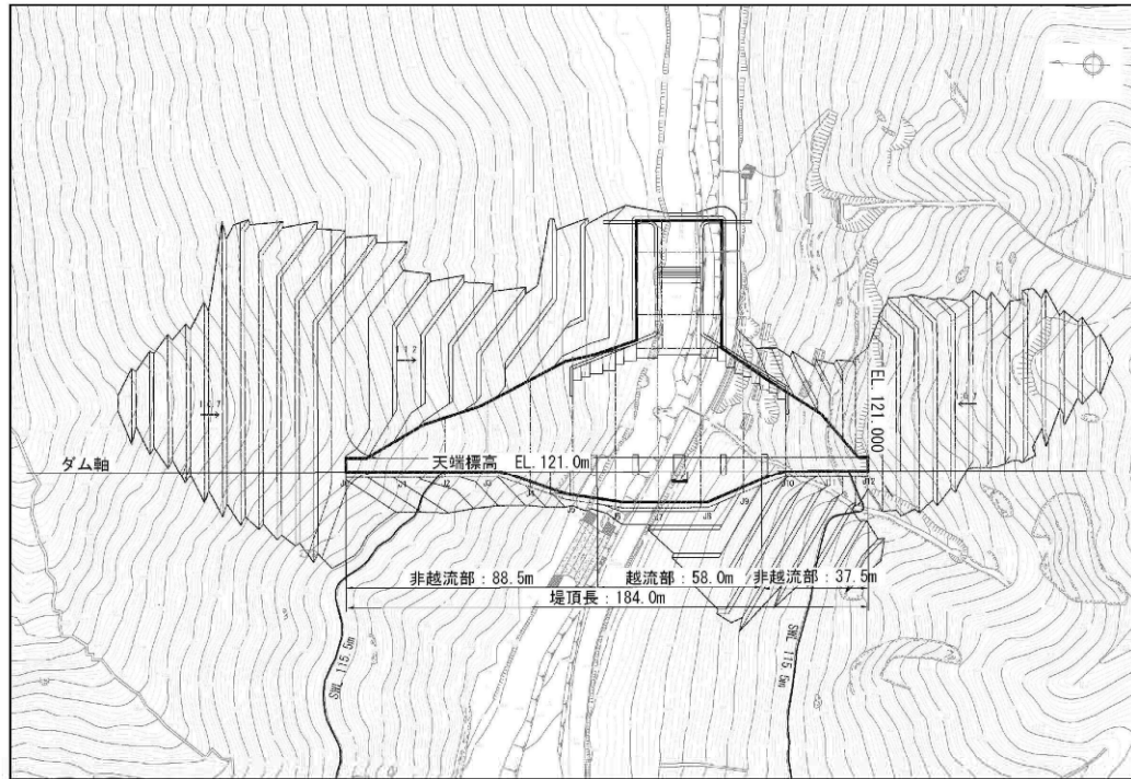
図 5.27 平面図
