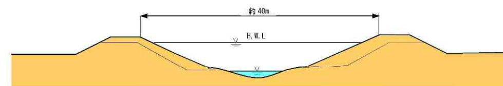
図 5.24 横断面図 (イメージ)
