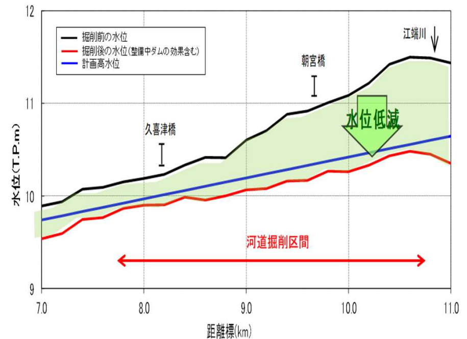
日野川における三尾野区間における河道掘削の概要
