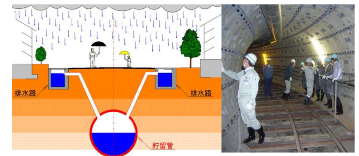
調整池以外の整備事例(月見・みのり雨水貯留管)
