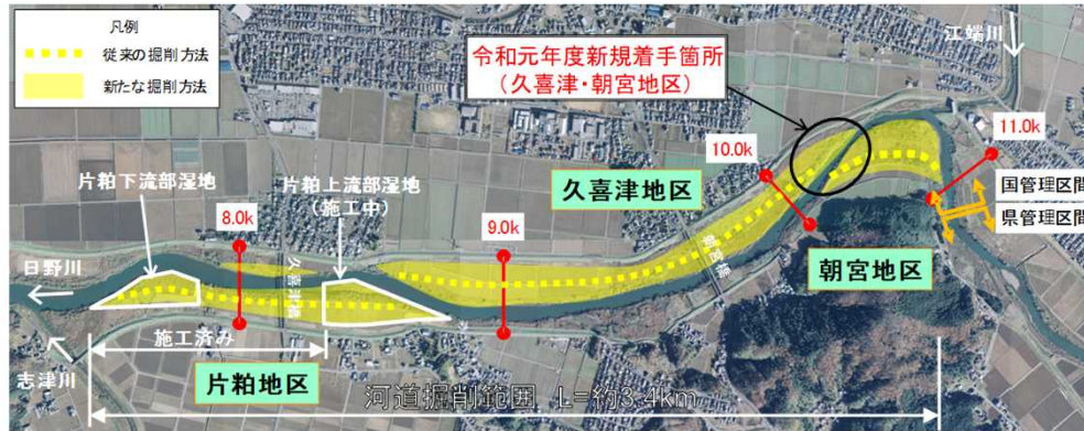
流下能力区間における河道掘削の例
