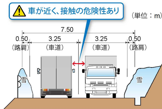
現況断面図
