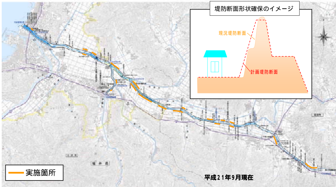
図 4.1.5 堤防断面形状確保実施予定箇所
