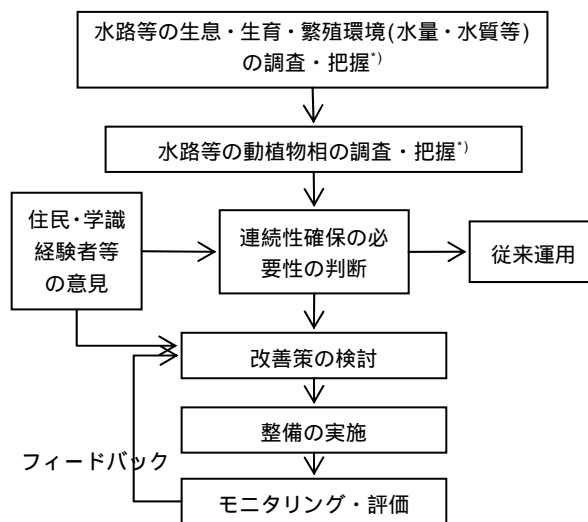
図 4.1.11 水路等との連続性確保対策フロー
