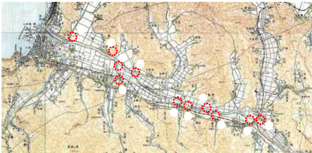
霞堤位置図
