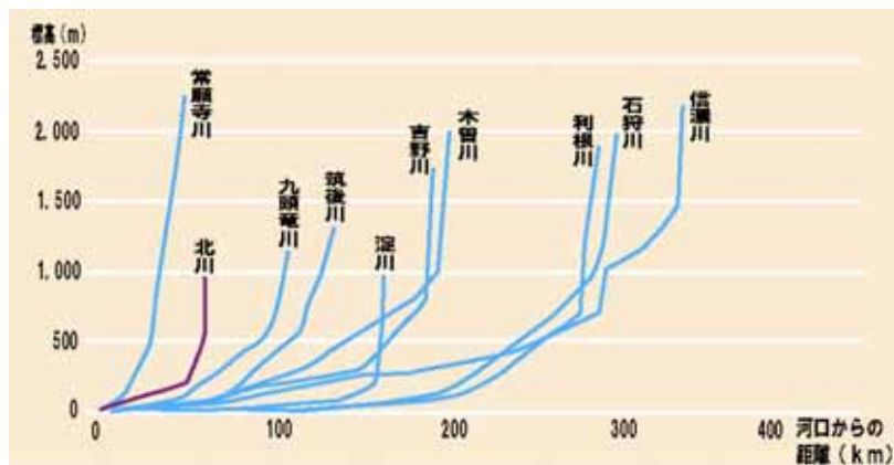
図 1.1.3 主要河川の河床勾配モード図
