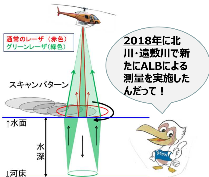
(航空機による測量のイメージ)
