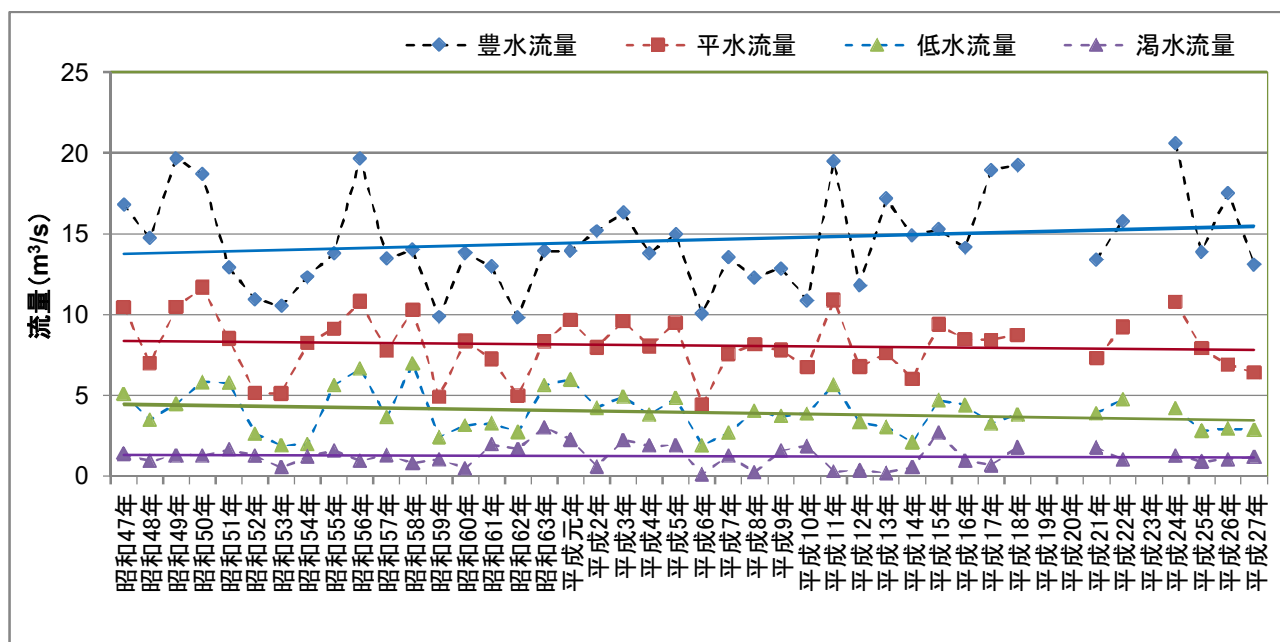
図 1.5.4 流況経年変化 (高塚地点)
