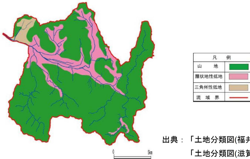
図 1.3.1 北川流域の地形区分
