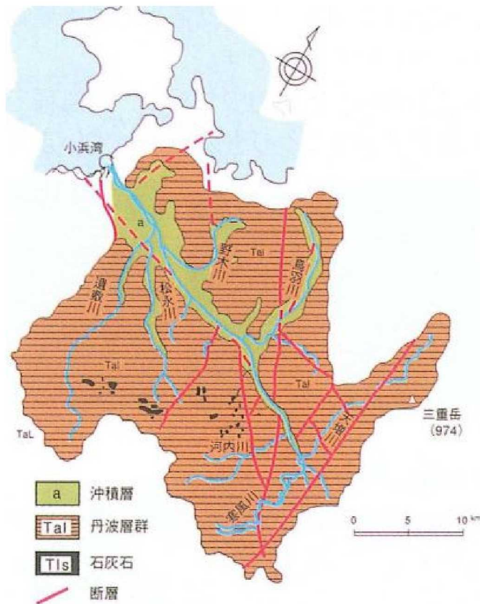
図 1.3.2 北川地質図 (出典：「北川改修30年史」平成15年)
