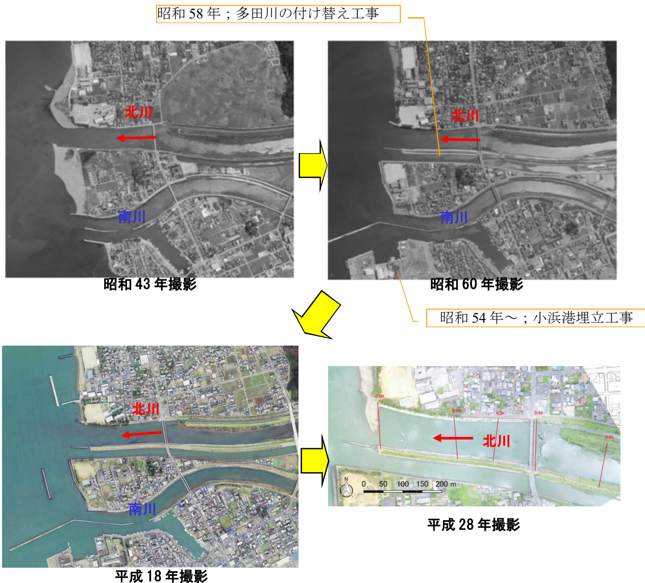
図 1.4.1 北川河口部の河道形状の経年変化
