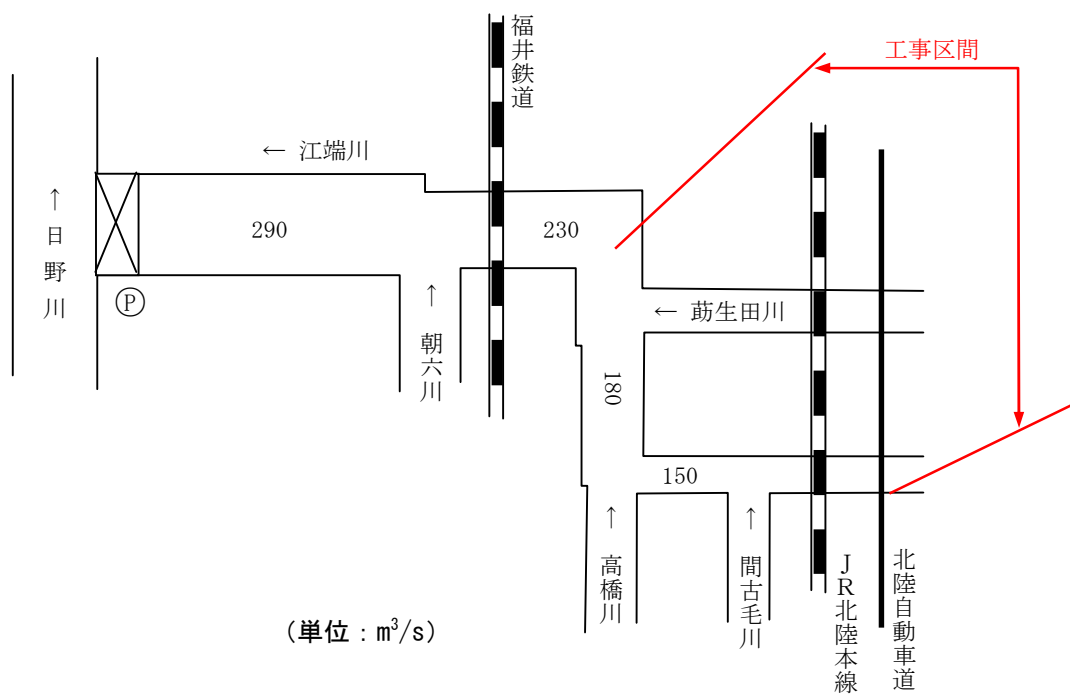
図 5.9 計画流量配分図
