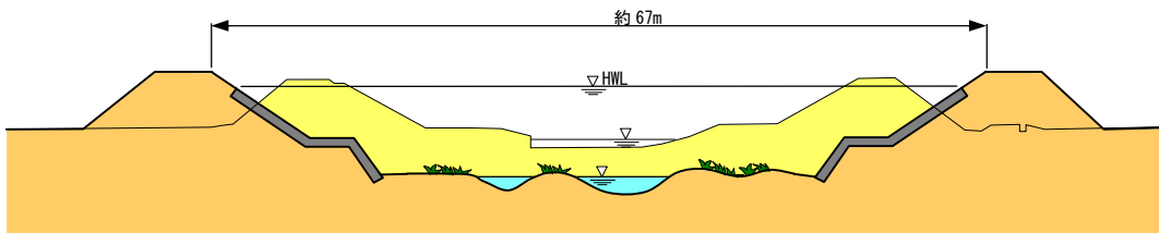
図 5.14 横断図 (イメージ)
