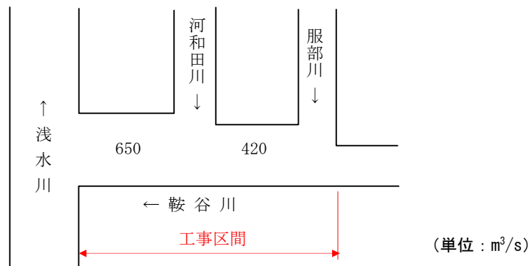
図 5.12 計画流量配分図
