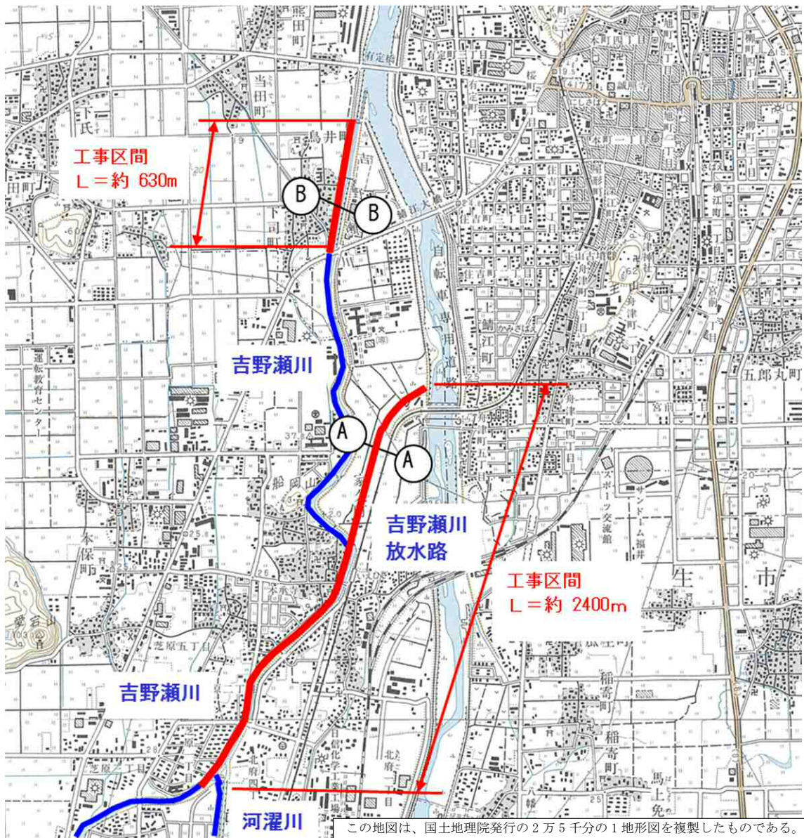
図 5.29 平面図
