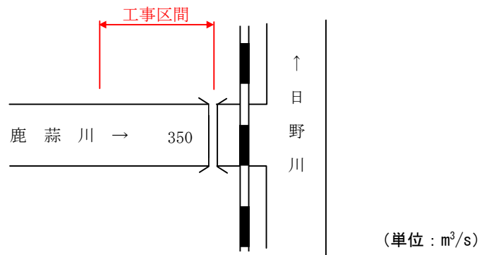
図 5.31 計画流量配分図
