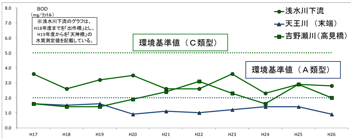
図 3.2 支川の水質 (BOD75%値) の推移
