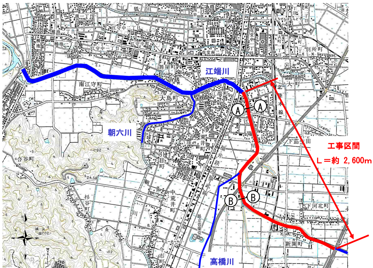
図 5.10 平面図
