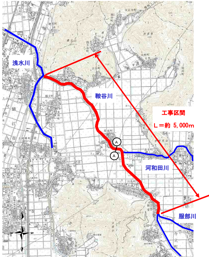
図 5.13 平面図
