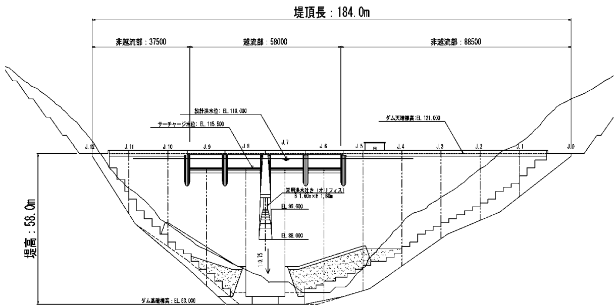
図 5.28 下流面図
