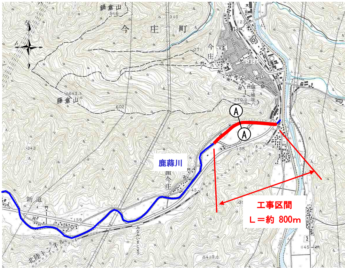
図 5.32 平面図
