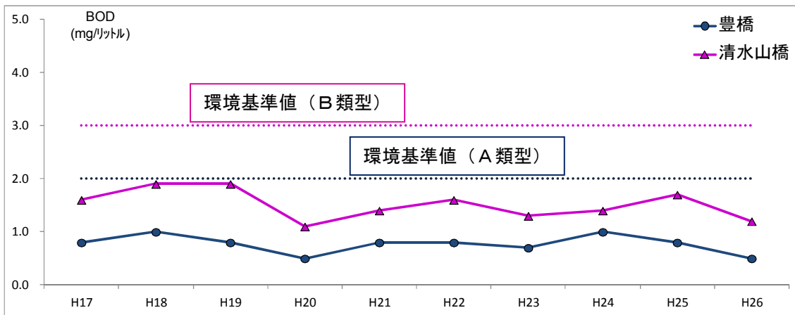
図 3.1 日野川の水質 (BOD75%値) の推移
