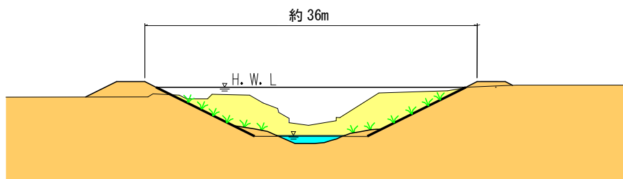
図 5.11 横断面図 (イメージ)
