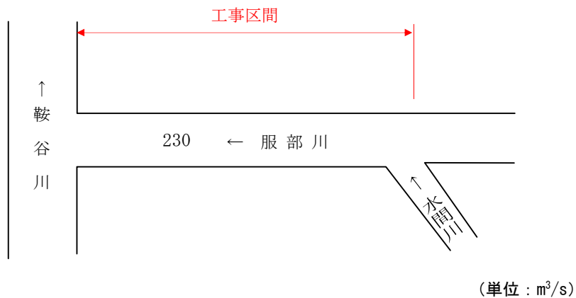
図 5.18 計画流量配分図
