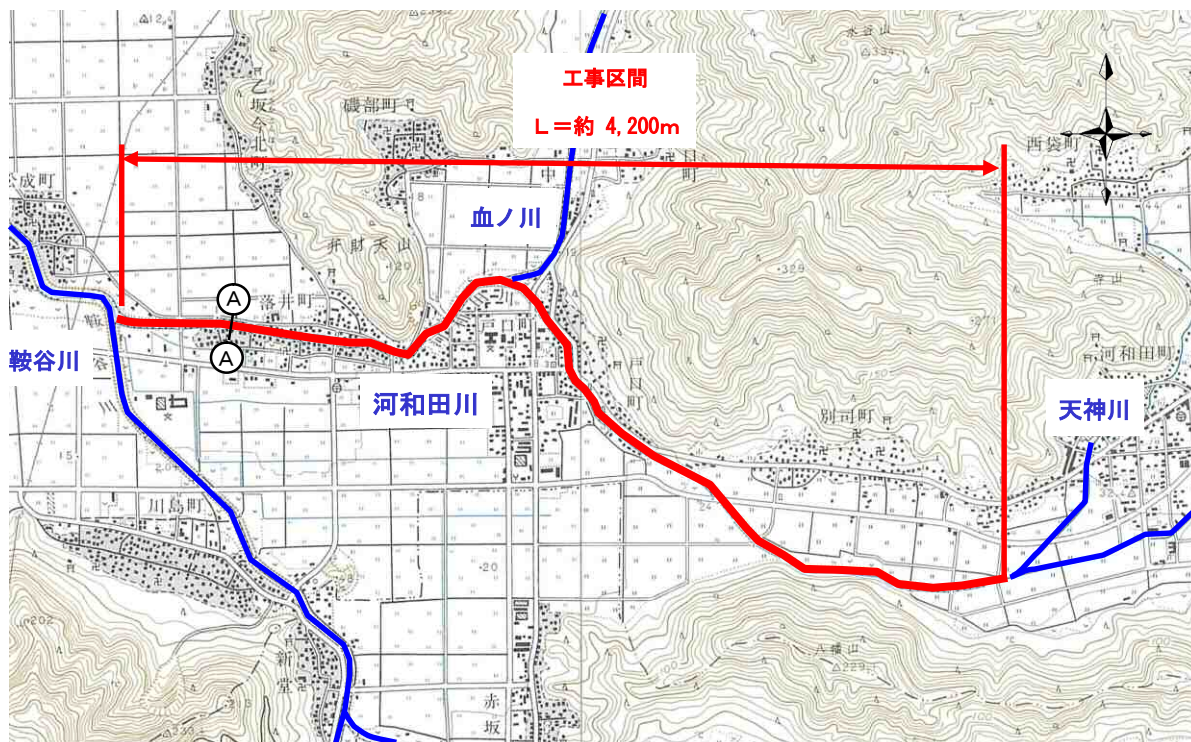
図 5.16 平面図
