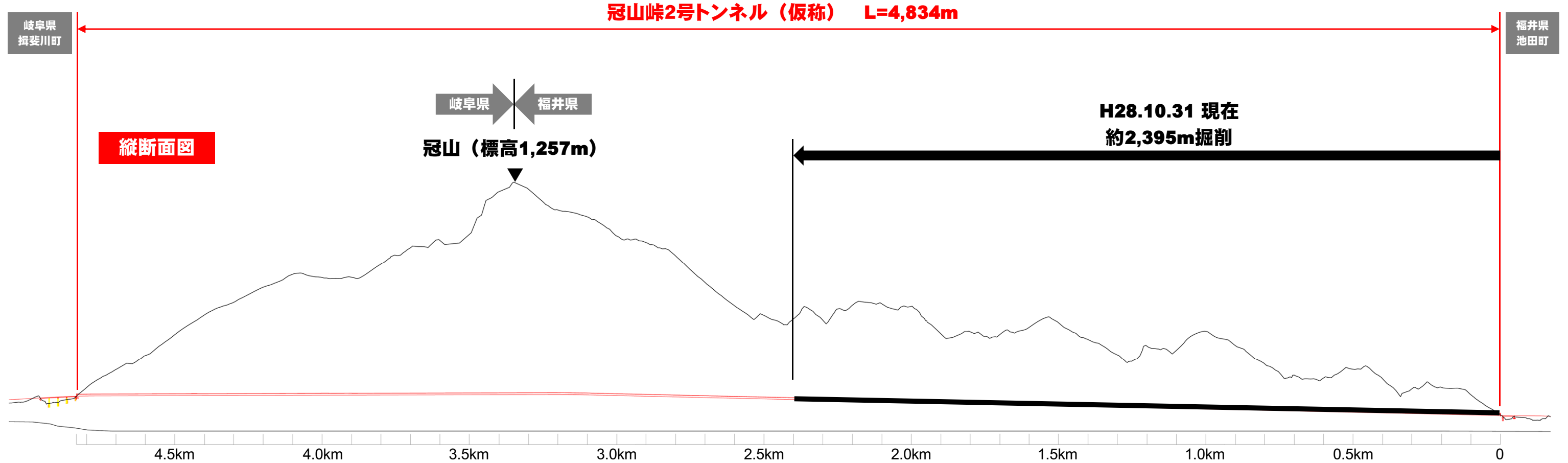
切羽の状況 (H28.10.31 撮影)
