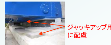
支保交換が容易な構造の例
