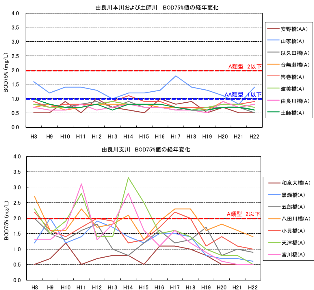
図 2.3.2 水質の経年変化 (BOD 75%値)
