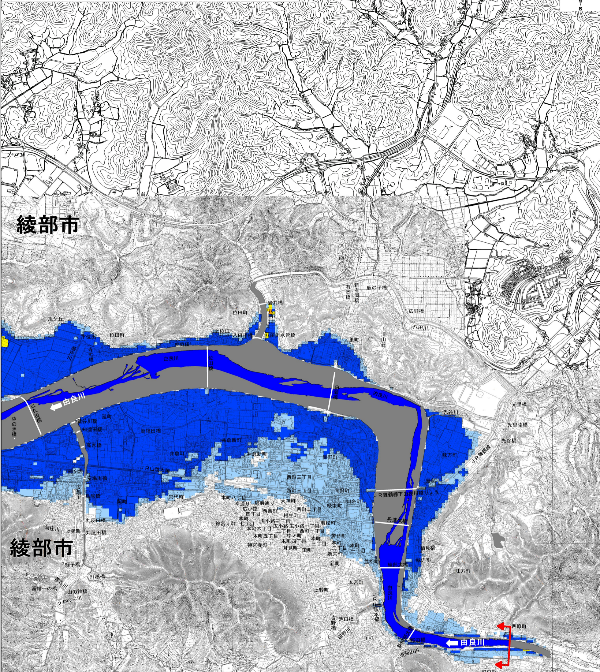
由良川水系由良川洪水浸水想定区域図 (浸水継続時間)
