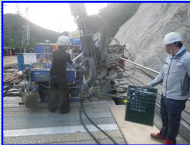
EPルートパイル施工状況
