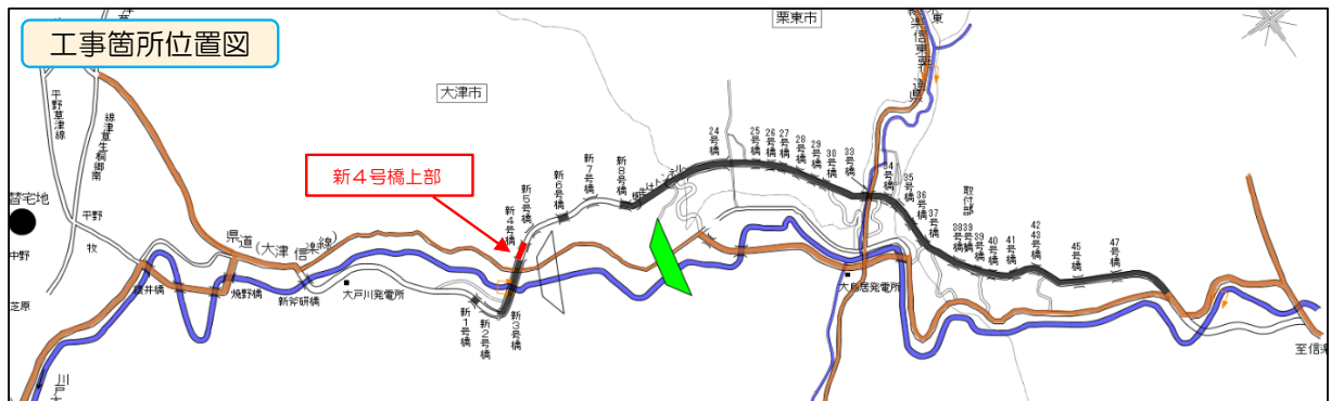
現場位置図
