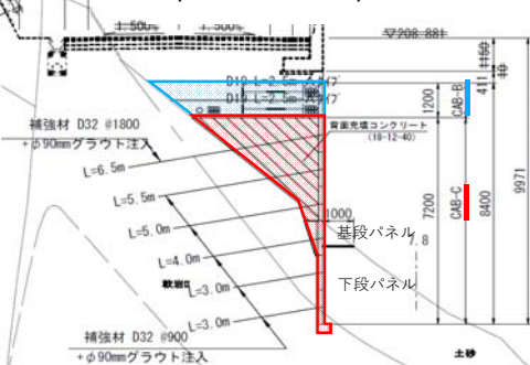
6号補強土壁工（CABWALL工法）
