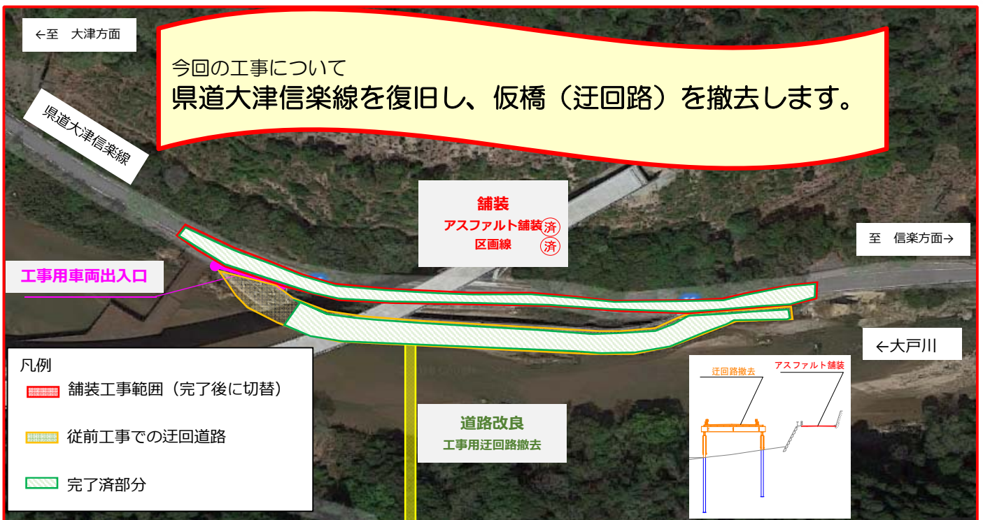
仮橋撤去開始！
