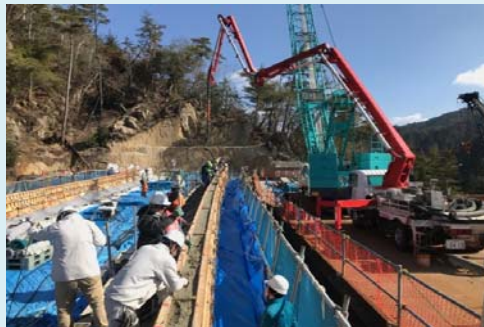
壁高欄コンクリート打ち込み状況
