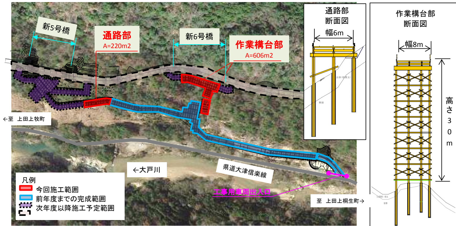
【 平面図 】
