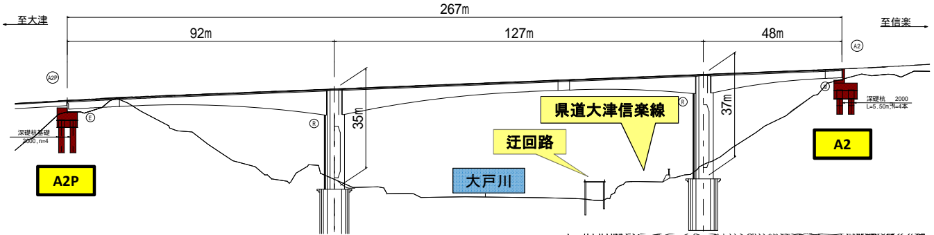
全体平面図
