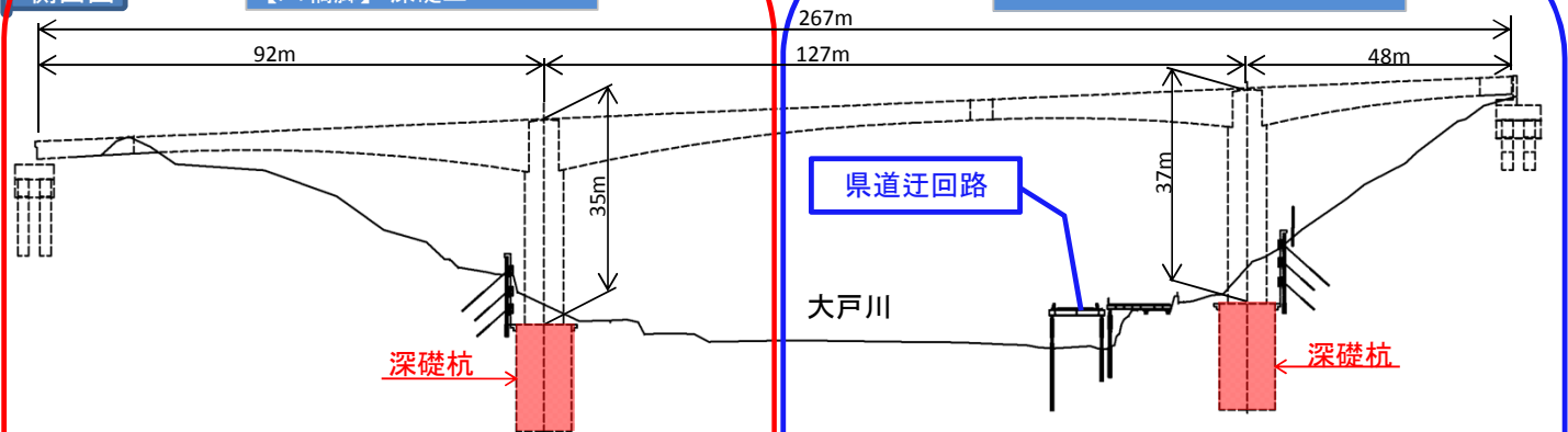
【P2橋脚】 深礎工
