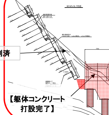
【A2橋台】(大戸川右岸部)
