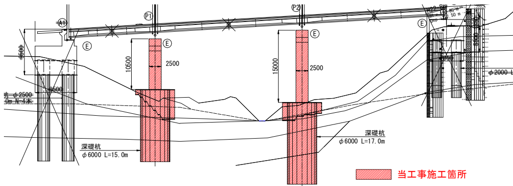
【工程表】
