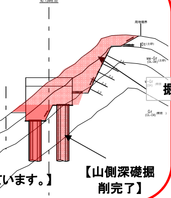
【A2P橋脚】(大戸川左岸部)
