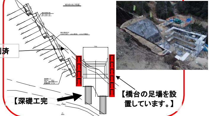
【A2橋台】(大戸川右岸部)
