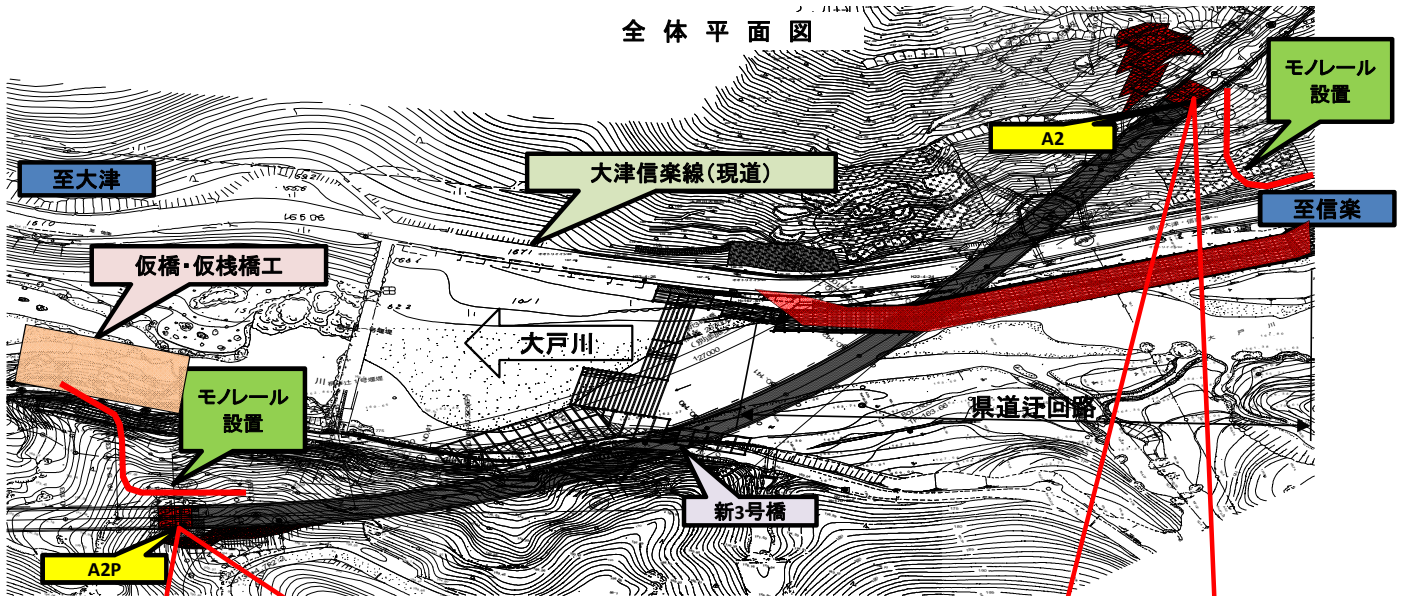
【A2P橋脚】(大戸川左岸部)
