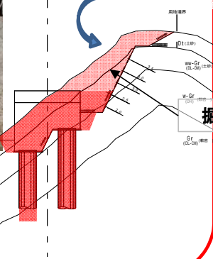
【山の斜面を掘削しています。】
