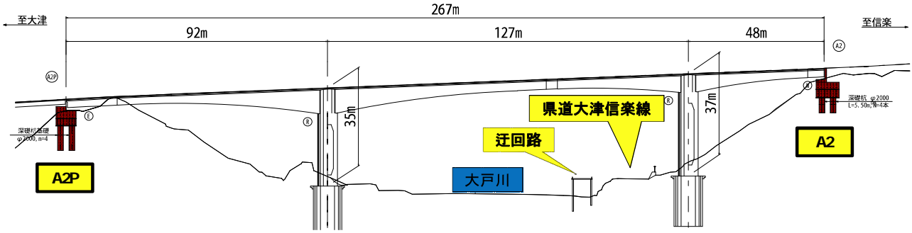
全体平面図
