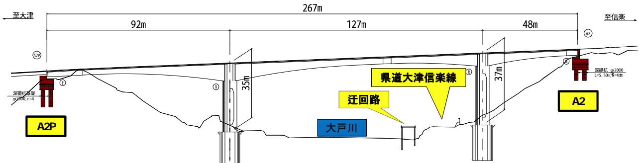
新3号橋 全体側面図
