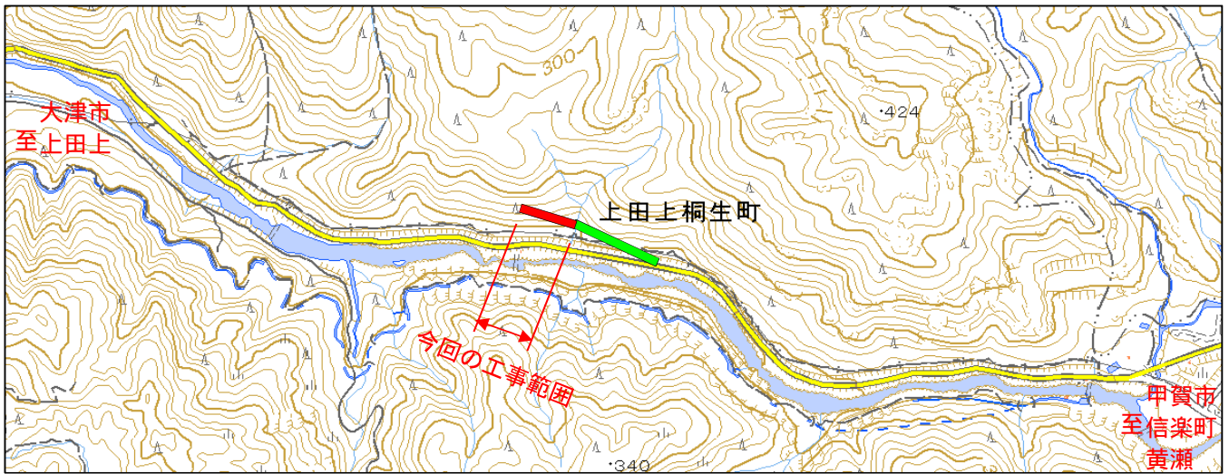
計画平面図
