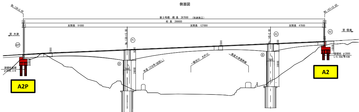
新3号橋全体側面図
