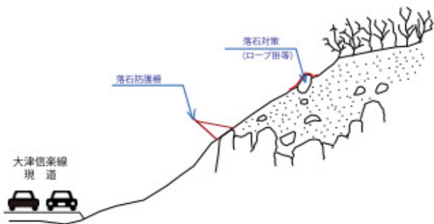
落石対策工 施工概要図
