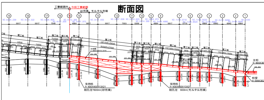
計画断面図
