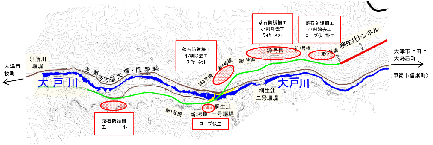
落石対策工 施工概要図
