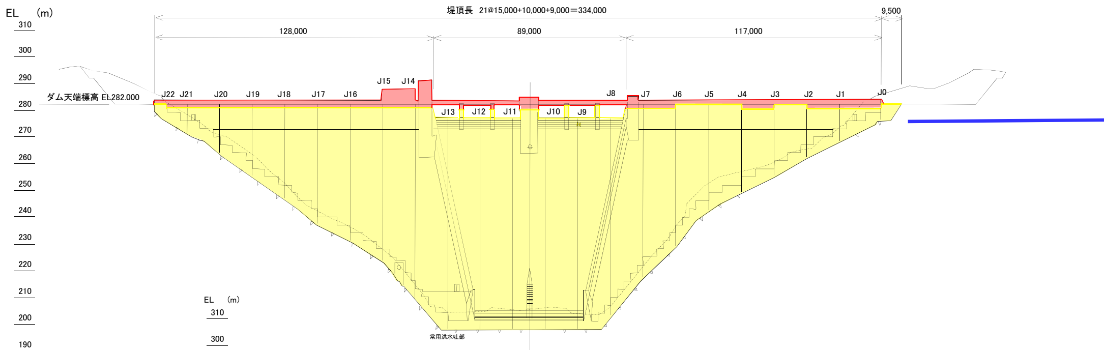
標準断面図
