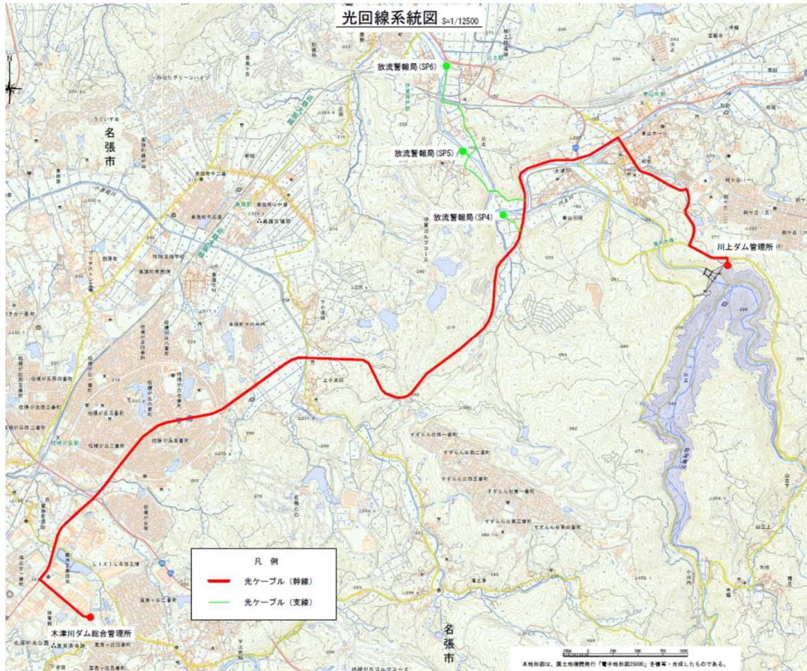
光ケーブル敷設経路
