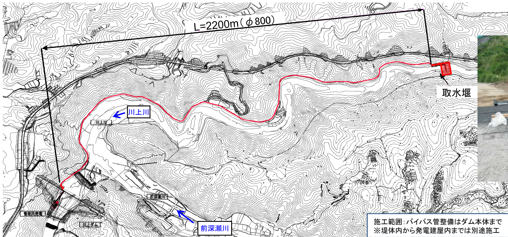
バイパス管施工状況
