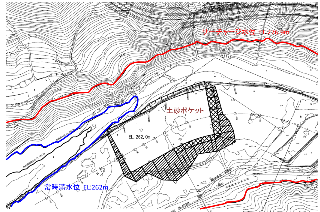
土砂ポケット平面図
