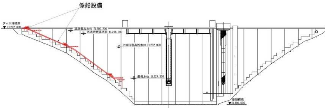
係船設備正面図
