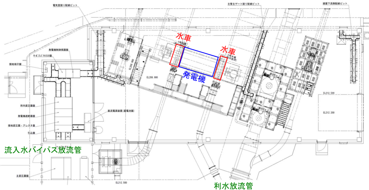
平面図
