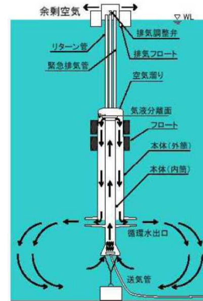
深層曝気設備イメージ(比奈知ダム)
