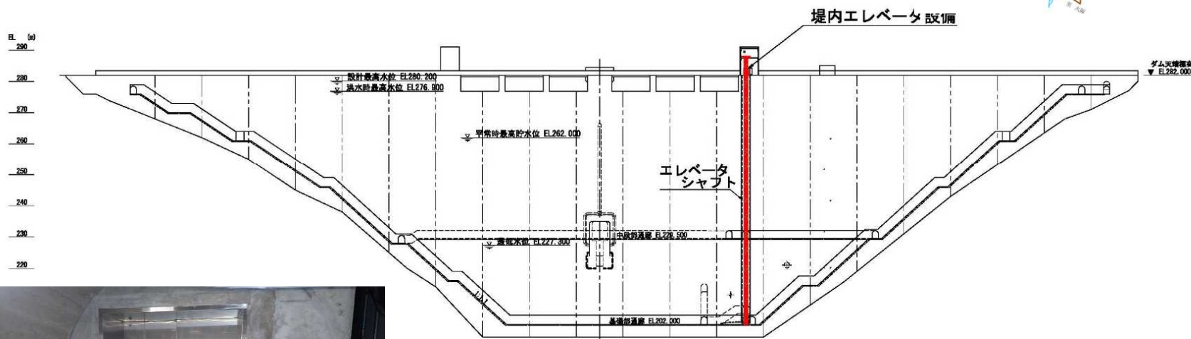
堤内エレベータ設備正面図
