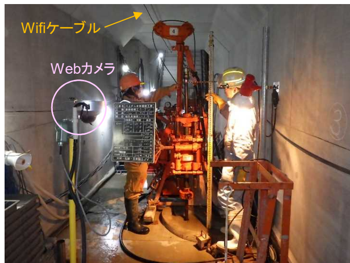
監査廊内wifi設置状況
