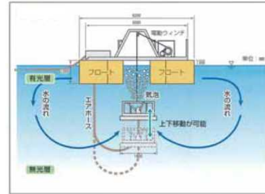
浅層曝気設備イメージ(小石原川ダム)
