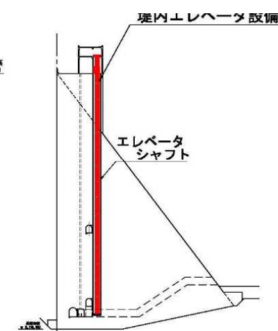
堤内エレベータ設備断面図
