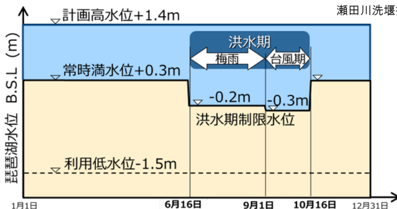
琵琶湖の水位管理図
