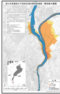
瀬田川下流洪水浸水想定区域図 (想定最大規模)
