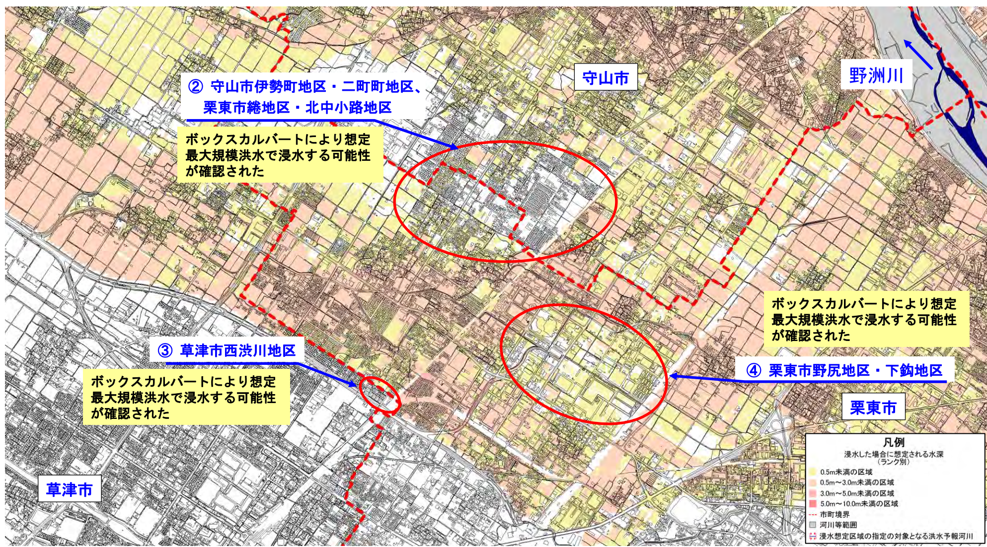
淀川水系野洲川洪水浸水想定区域図（想定最大規模降雨）（平成28年6月公表）抜粋
