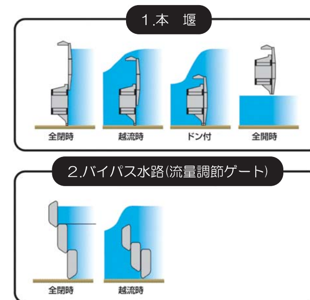
ゲート操作図
