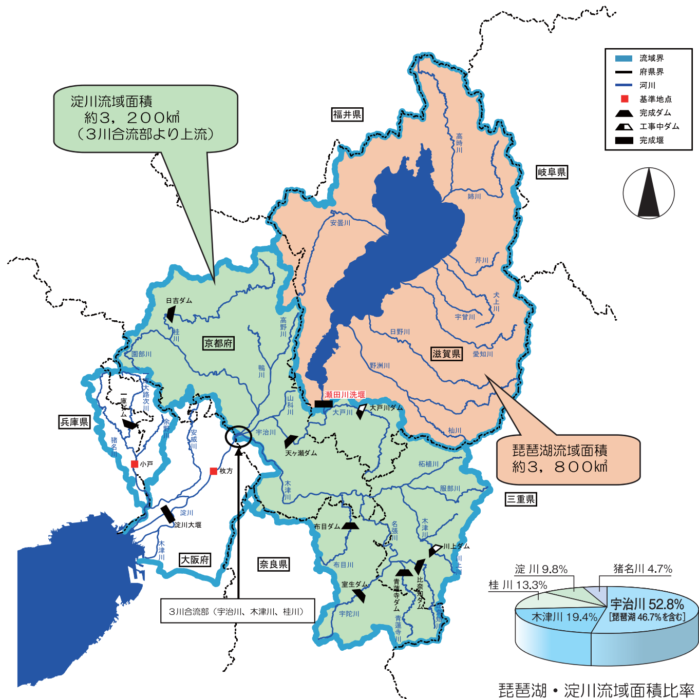
淀川水系の流域図
