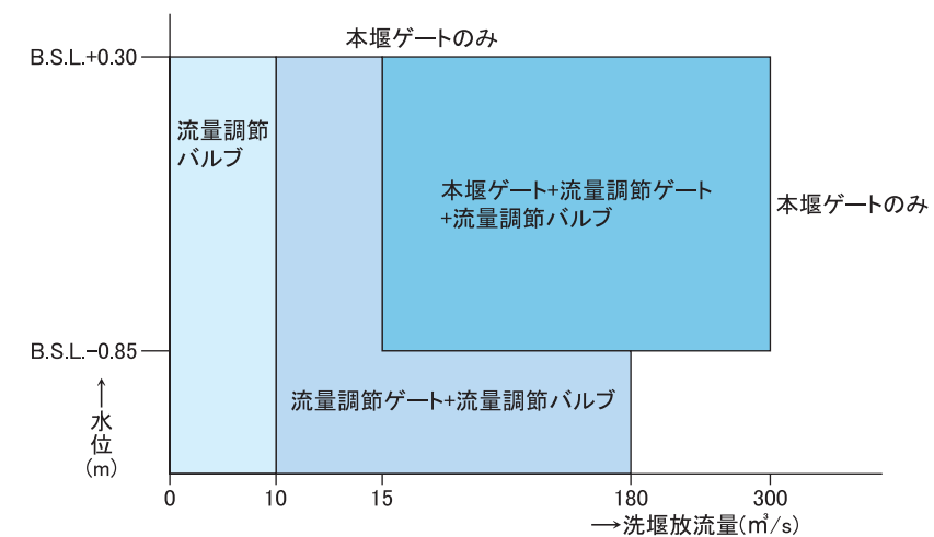
放流分担図
