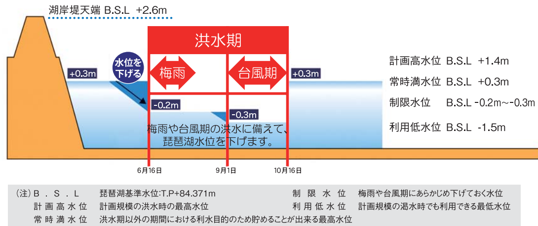
琵琶湖の水位管理図及び水位移行時の操作
