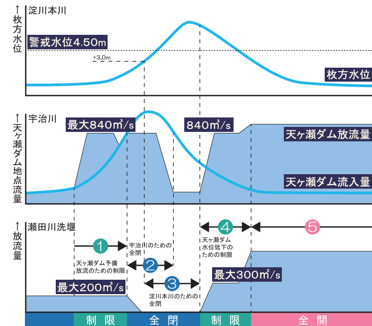
洪水時の操作概念図
