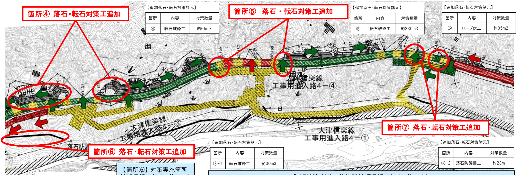
【追加落石・転石対策諸元】
