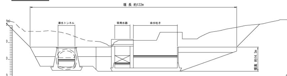
下流面図
