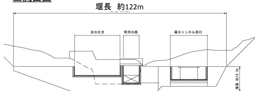
上流面図
