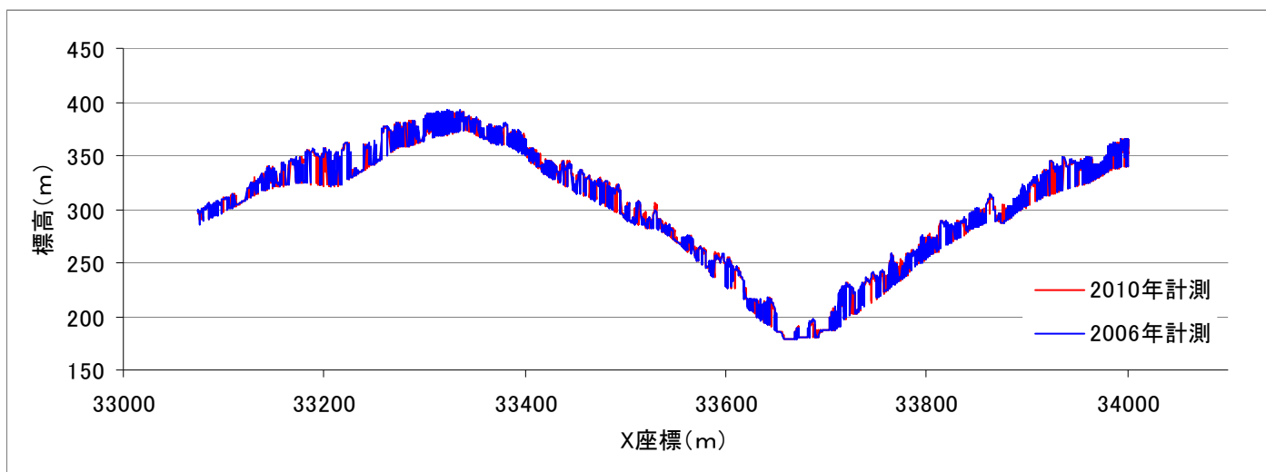
ダムサイトの断面図による比較 (A-A')
