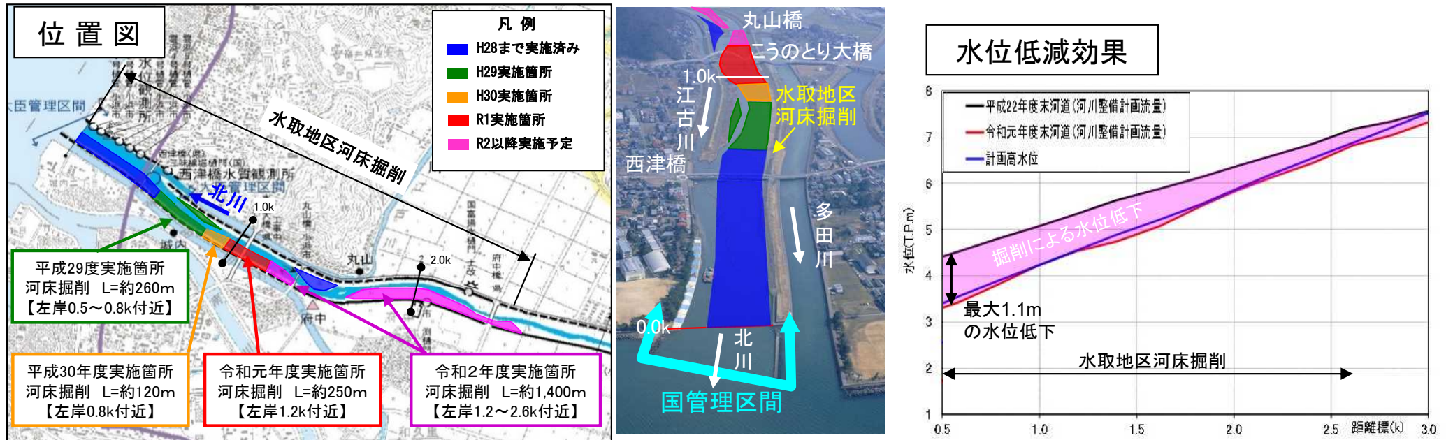
北川の下流域における河道掘削の概要
