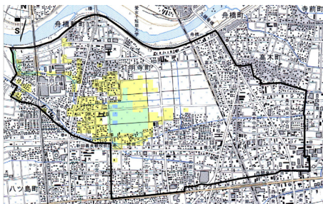
【事業前】旧馬渡川樋門+河川改修前
