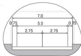
標準断面図 トンネル部
